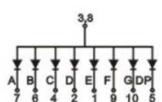
PCB:D5212A/B
