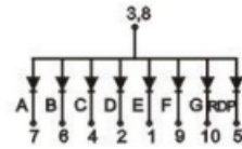
PCB:D3011E/F
