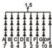
PCB:D23011A/B
