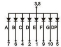
PCB:D10018A/B
